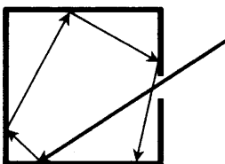
Модель абсолютно чёрного тела
